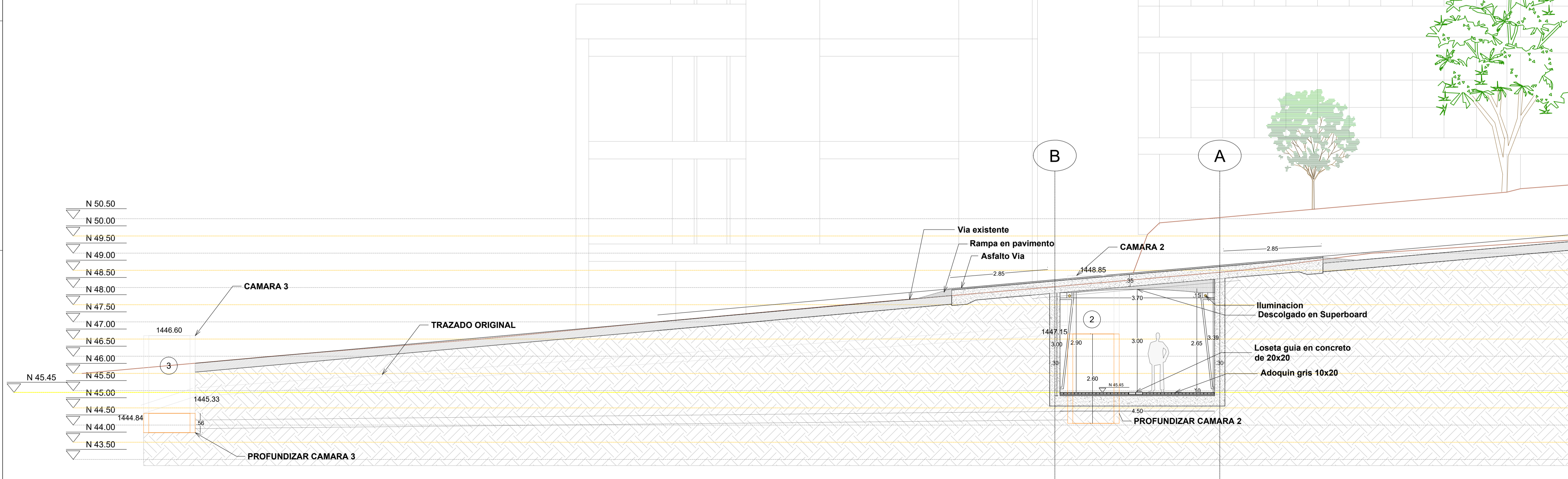
D12 4 Movimiento de cámaras 2-3 Esc 1:75
